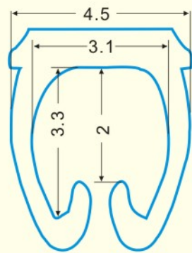
规格: 1.5mm 2
